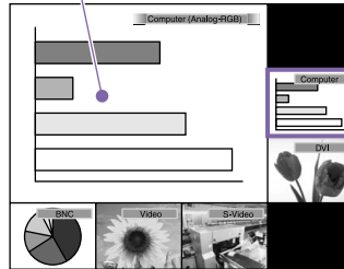
Aktives Fenster
