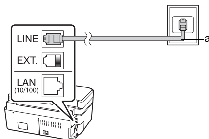
a Mufa telefonică de perete
