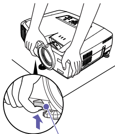
Languelette de réglage du pied
