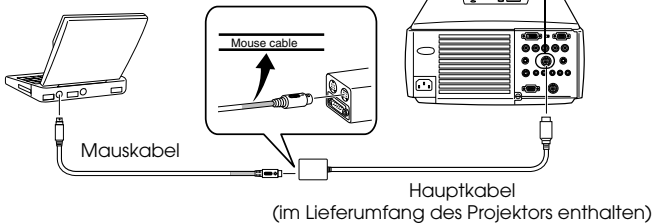
PS/2-Anschluss
