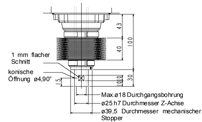
Detail von "A" (Position der Kalibrierungspunkte der 3. und 4. Achse)
